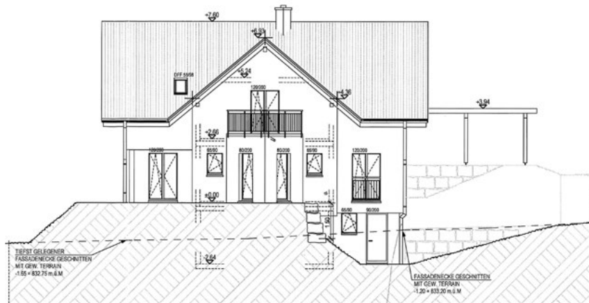
Südfassade
