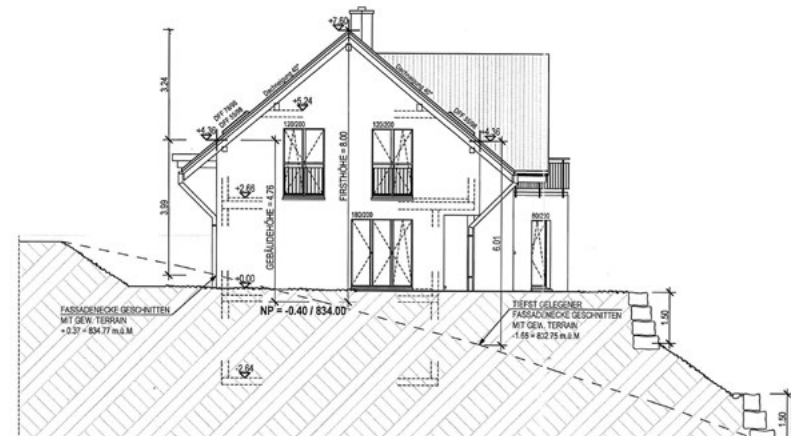
Westfassade
